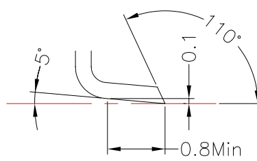
DETAIL:A-10:1 PATENTED
